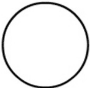
Uranus
